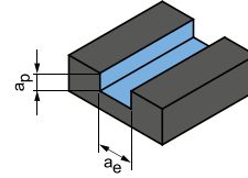
Groove milling
