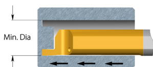
Face Grooving
