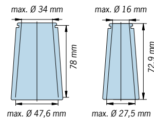
Für Kühlkörper / For Cooling body: Ø 25–32 mm Ø 14–16 mm
