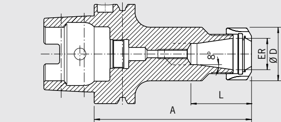
Kühlmittelrohr auf Wunsch/Coolant tubes on demand
