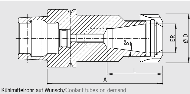
Kühlmittelrohr auf Wunsch/Coolant tubes on demand
